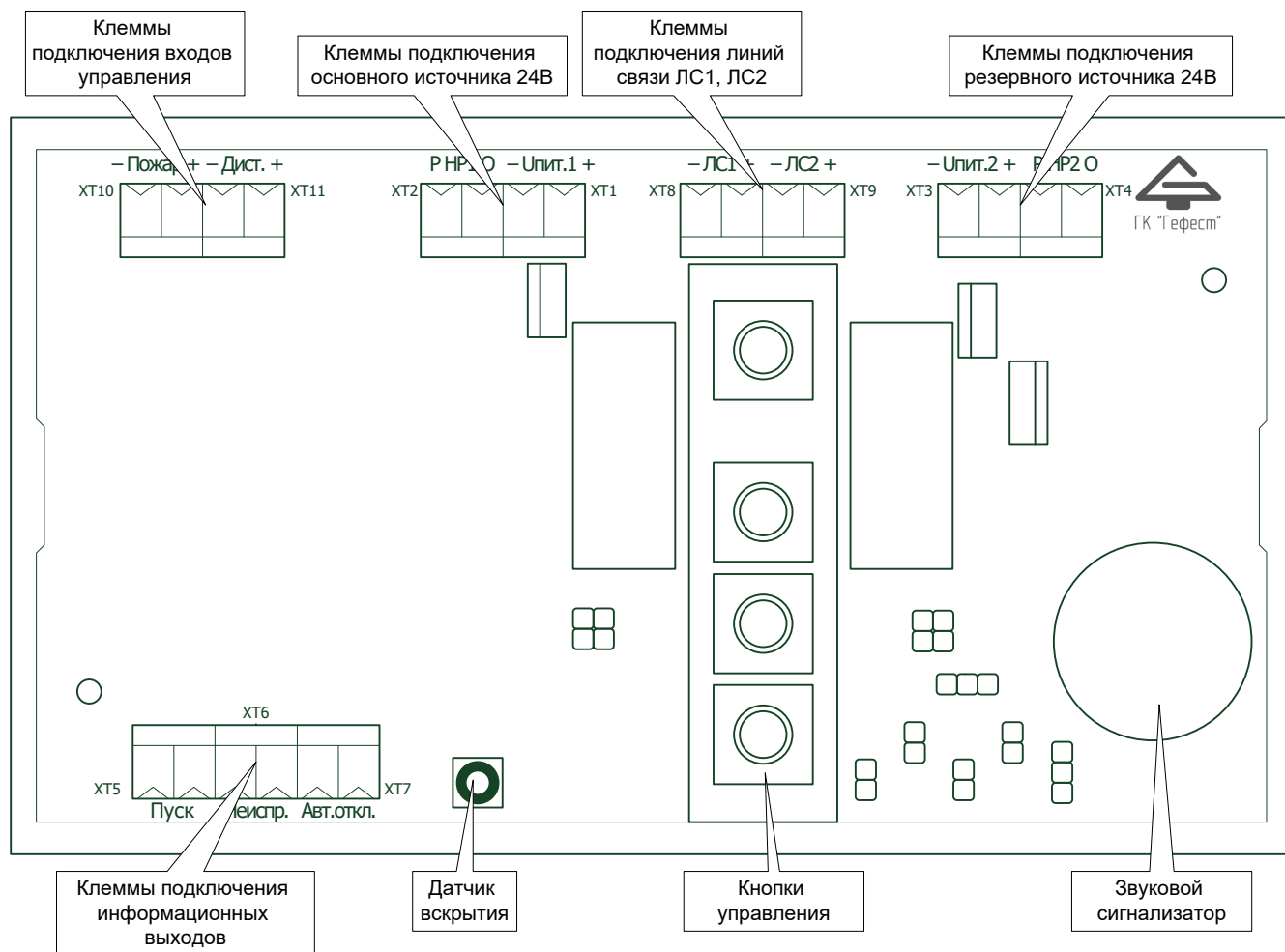
Рисунок 2. Плата ЦБ.
